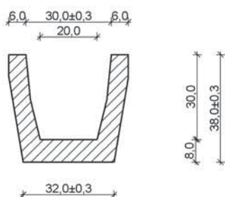
keresztmetszet
