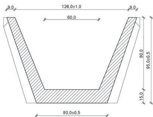
keresztmetszet
