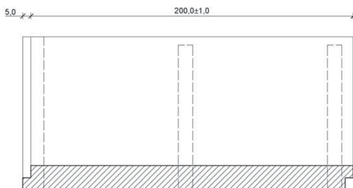
hosszmetszet
