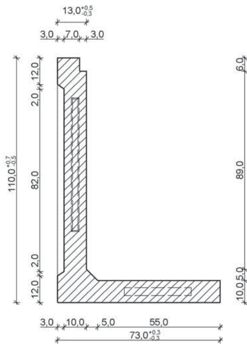
keresztmetszet
